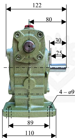
Input Shaft
