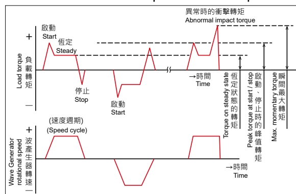
負載轉矩模式範例 Example of Load Torque Pattern
