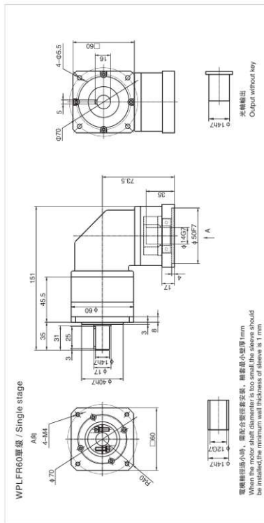
WPLFR60精密行星減速機外形圖 /
