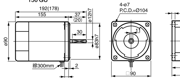
⑯ 5RK 120 GN-□ 重量 3.4kg 90 A 150 GU
