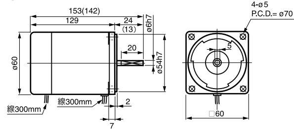
① 2IK6A(GN)-□B 重量 1.2kg
