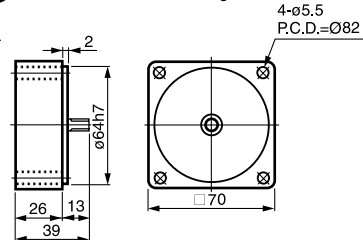
⑥ 3GN-10X 重量 0.35kg
