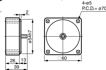
③ 2GN-10X 重量 0.3kg
