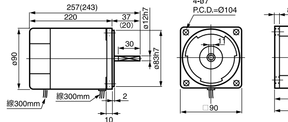
⑯ 90 A 5IK 120 GN-□ 150 GU 重量 4kg
