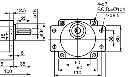
⑰ 5GU-3~180 K 重量 1.3kg (60, 90, 120, 150W 共用)
