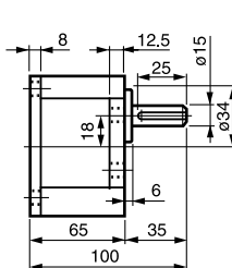
⑪ 5GU-3~180 K 重量 1.3kg (60, 90, 120, 150W 共用)
