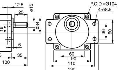
⑰ 5GU-3~180K 重量 1.3kg (60, 90, 120W 共用)
