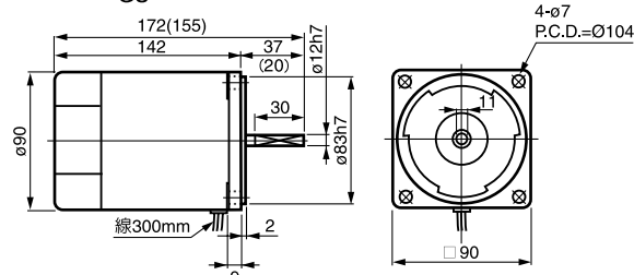
⑬ 5RK60 GN-□ 重量 2.6kg 90 A GU
