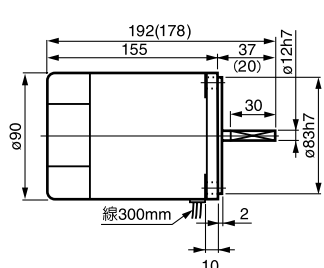
⑩ 5IK 120 GN - □ / 5IK 150 GN - □ 重量 3.4kg GU GU
