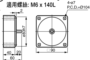
⑮ 5GU-10XK 重量 0.65kg
