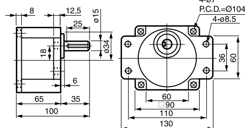
⑰ 5GU-3~180 K 重量 1.3kg (60, 90, 120, 150W 共用)
