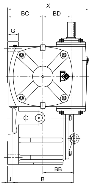
VOH155~175
