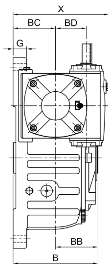
VOH60~135
