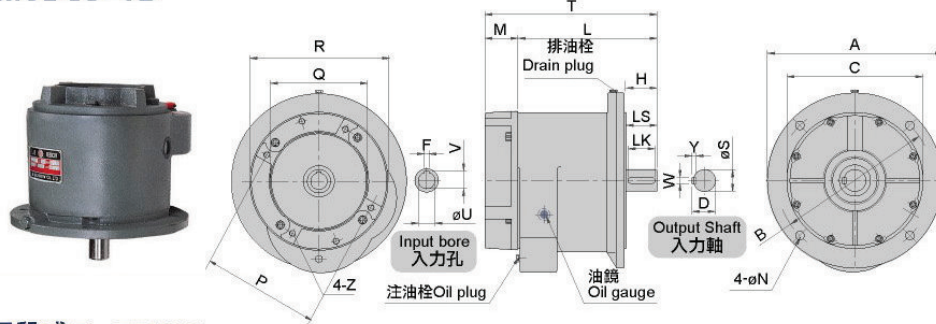
尺寸表 Dimension
